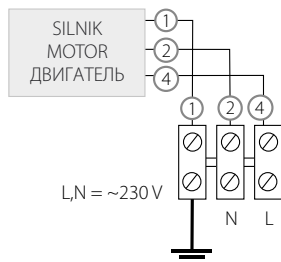
SCHEMAT PODŁĄCZENIA CONNECTION SCHEME / СХЕМА ПОДКЛЮЧЕНИЯ WB-5
