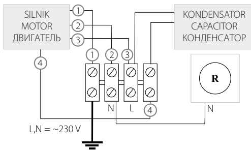
SCHEMAT PODŁĄCZENIA CONNECTION SCHEME / СХЕМА ПОДКЛЮЧЕНИЯ REGULATOR OBROTÓW / SPEED CONTROLLER / РЕГУЛЯТОР ОБОРОТОВ WOS, WOKS (Ø200-Ø630)
