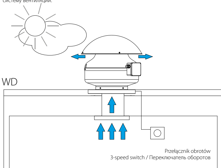
WD Montaż dachowy - wyciąg na zewnątrz budynku przy zastosowaniu zestawu montażowego. Roof installation - exhaust outside the building using the installation set. Монтаж на крышу - вытяжка наружу здания при помощи монтажного набора.
