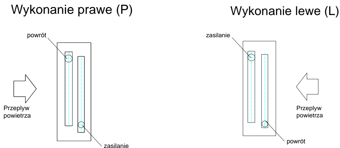
Rys. 3.6 Sposób podłączenia wymiennika wodnego a) wykonanie prawe, b) wykonanie lewe
