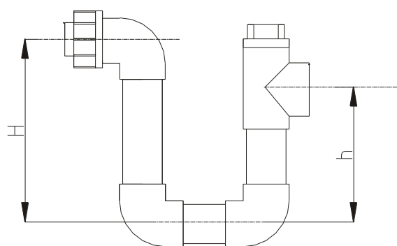
Rys. 3.7b Syfon sekcji pracujących na nadciśnieniu
