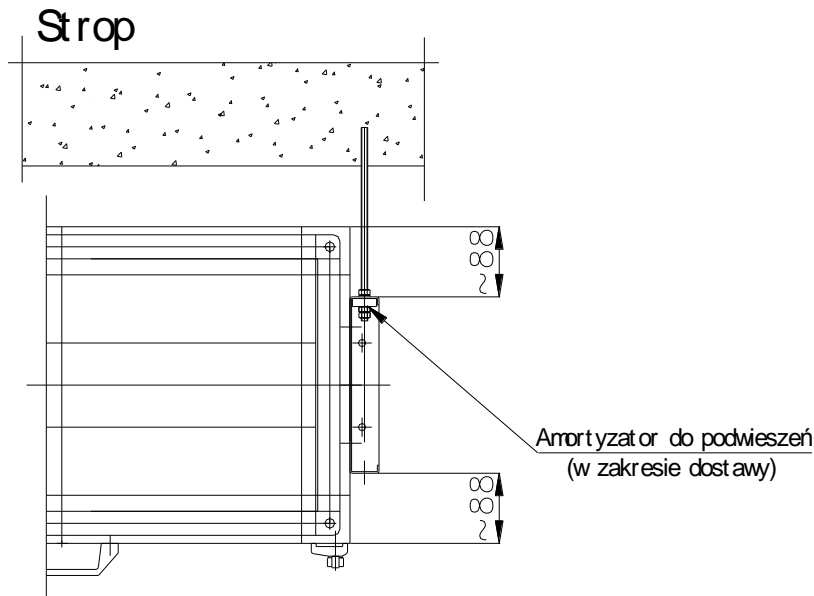
Rys. 3.1 Montaż centrali w pozycji podwieszanej
