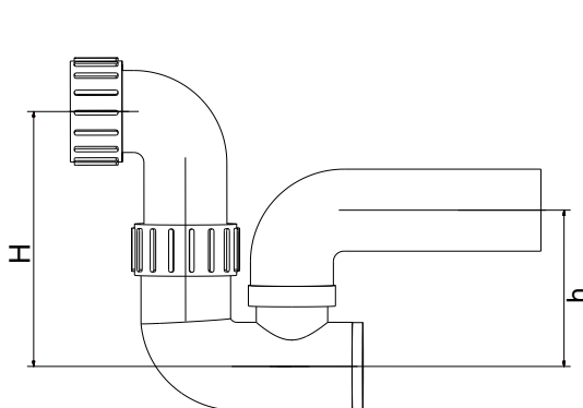
Rys. 3.7a Syfon kulowy
