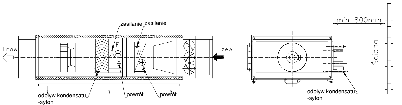
Rys. 1.1 Strona wykonania central oraz jej lokalizacja
